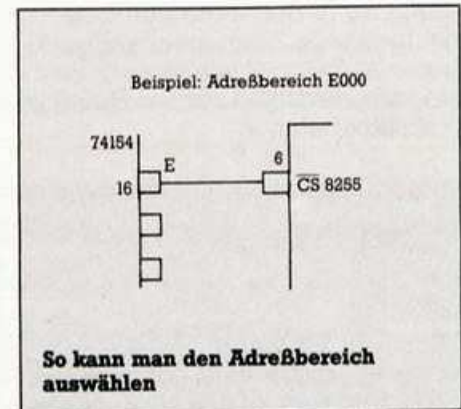
Mit dieser Schaltung kann der Prommer an beliebige Computer angeschlossen werden
