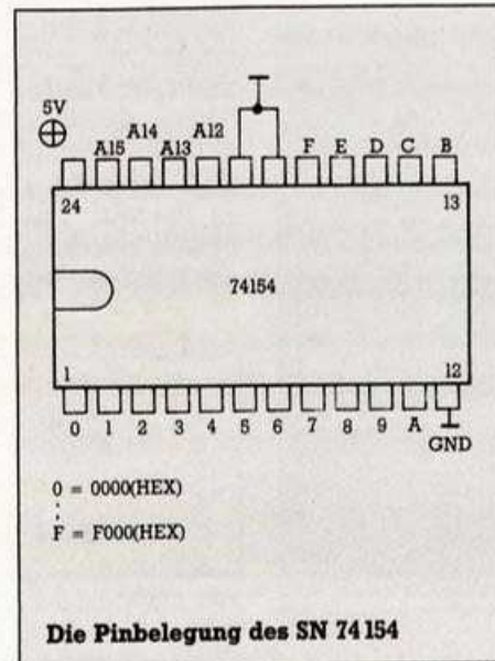
So wird der Prommer an den C 64 angeschlossen
