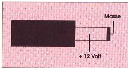
Der Anschluß des 12-Volt-Steckers am CPC-Monitor
