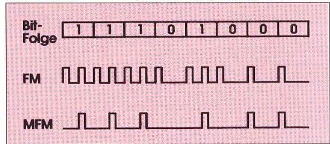
Oben: Das MFM-Verfahren ermöglicht gegenüber dem älteren FM-Verfahren die doppelte Aufzeichnungsdichte Links: Die Aufteilung der Diskette in Spuren und Sektoren Unten: Um die Vorgänge bei der Speicherung zu verdeutlichen, schreiben wir hier den Buchstaben S auf die Diskette
