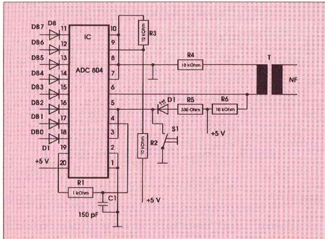
Die Schaltung des A/D-Wandlers
