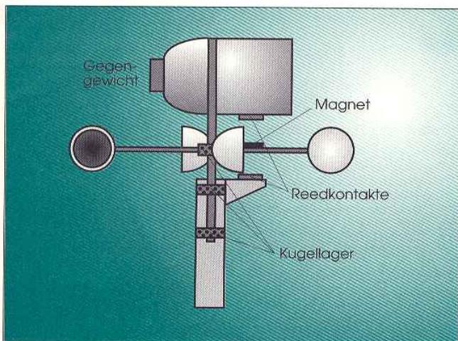
Abb. 2: Der Aufbau der Windrichtungs- und Stärkemessanlage beschränkt sich auf ein Minimum an Teilen
