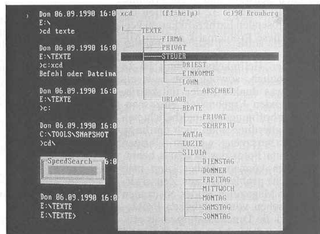
Der Verzeichnisbaum einer Festplatte, ausgegeben von XCD
