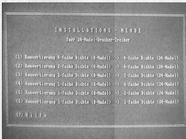
Bild 1: Das Anpassungs-Menü
