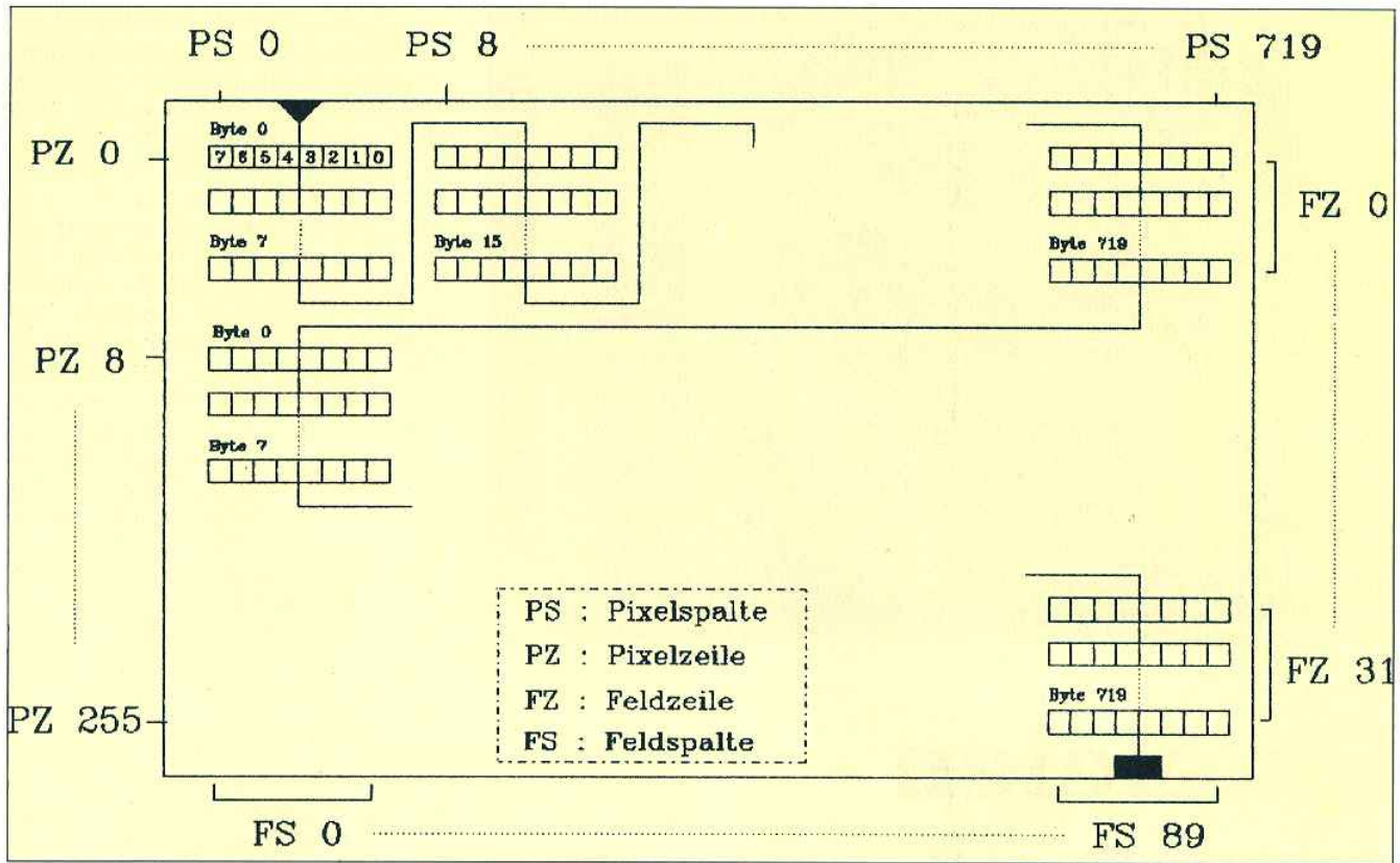
Abb1: Der Bildschirmaufbau des JOYCE im Überblick
