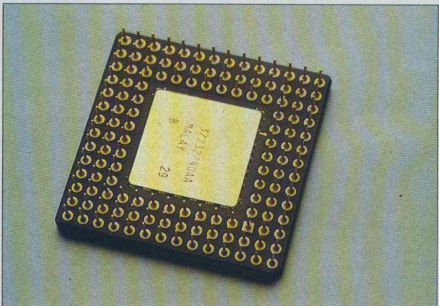
Abb.2: Das Herz des PC 2386: Der 80386-Prozessor. Mit seinem 32-Bit-Bussystem, den erweiterten Befehlen und einer speziellen Abarbeitung derselben macht er den PC2386 zu einem Rennpferd in der MS-DOS-Welt
