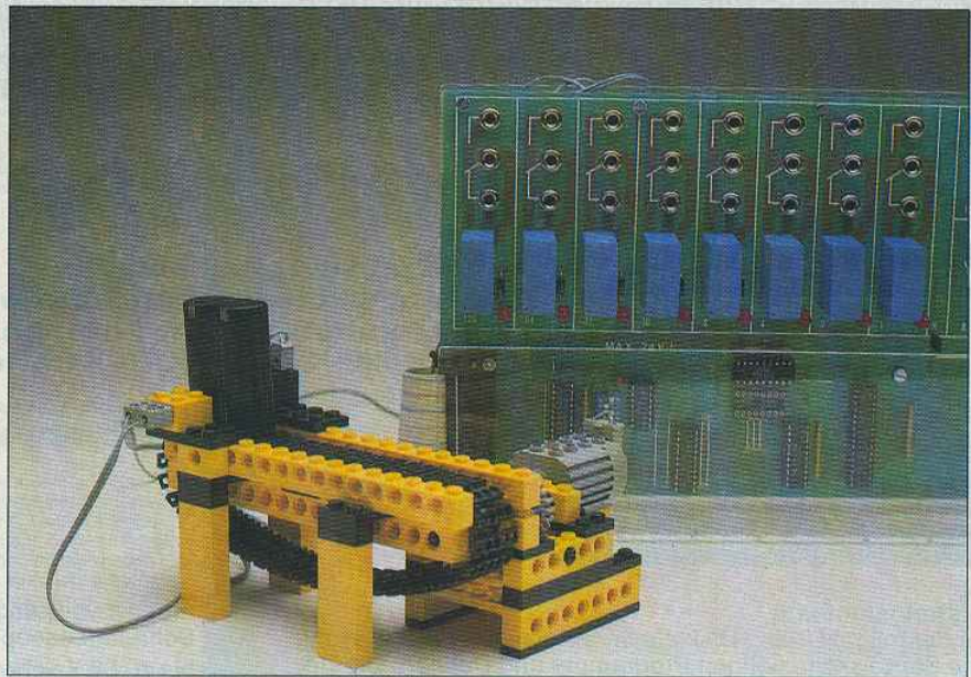
Abb 2: Nachdem der Gegenstand die Lichtschranke unterbricht, steht das Laufband still
