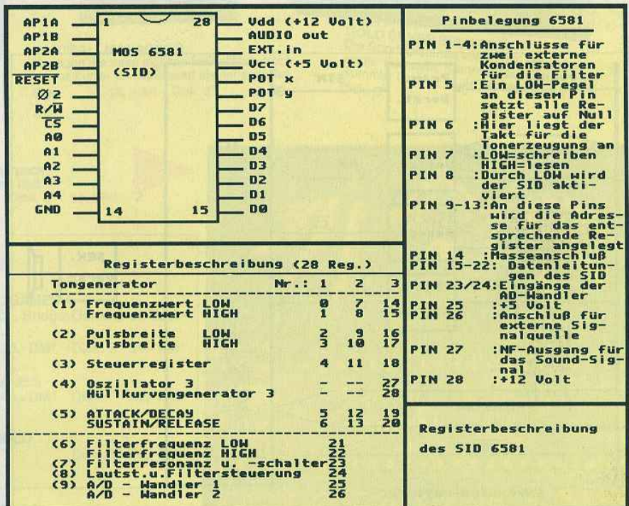
Abb. 2: Die Pinbelegung des MOS6581 mit der Registerbeschreibung
