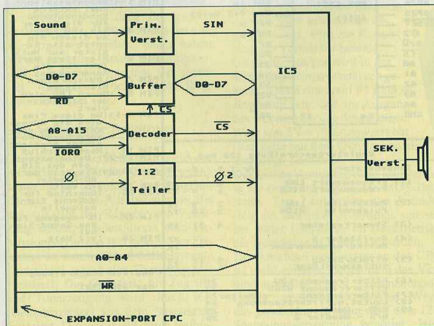
Abb.4: Das Blockschaltbild der gesamten Schaltung
