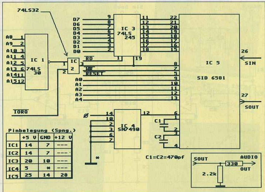
Abb. 1: Das Schaltbild für den Anschluß des Soundchips SID am CPC. Die Tabelle in der linken Ecke zeigt den Anschluß der Stromversorgung am jeweiligen IC an
