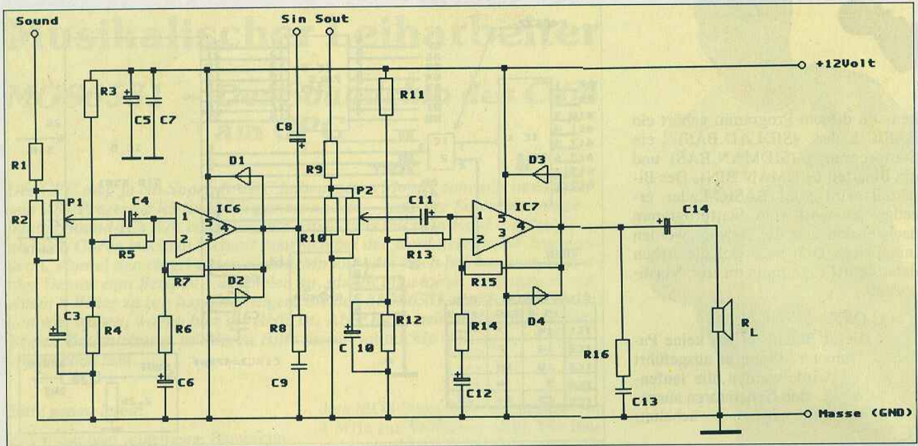
Abb.3: Der Schaltplan des Primär- und Sekundärverstärkers. Beide Verstärker-ICs sollten gekühlt werden
