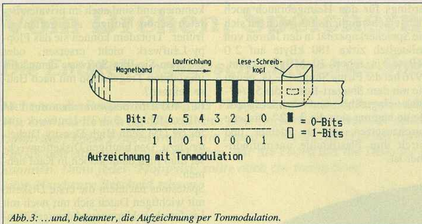
Abb.3: ...und, bekannter, die Aufzeichnung per Tonmodulation.
