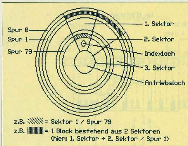
Abb.12: Der schematische Aufbau einer (formatierten) Diskette.
