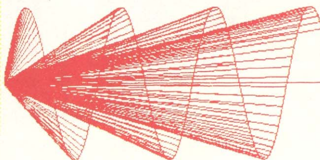
Drei-dimensionale Sinusfunktion, dargestellt im Koordinatensystem
