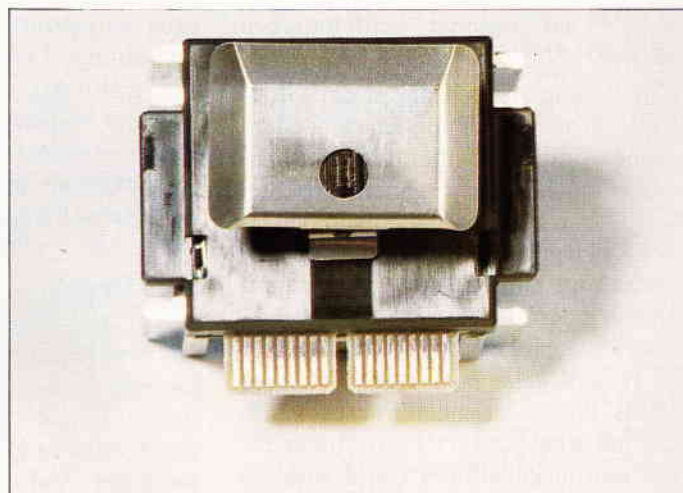
Bild 2: Der Nadeldruckkopf bildet ein Zeichen durch Punkte nach...
