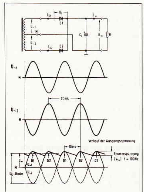
Bild 1a: Mittelpunktleitrichtung mit Spannungsverlauf
