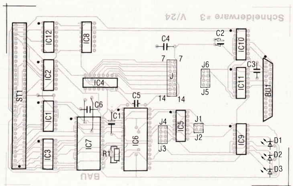
Bild 1: der korrekte Bestückungsplan der V/24 aus Heft 8/86.
