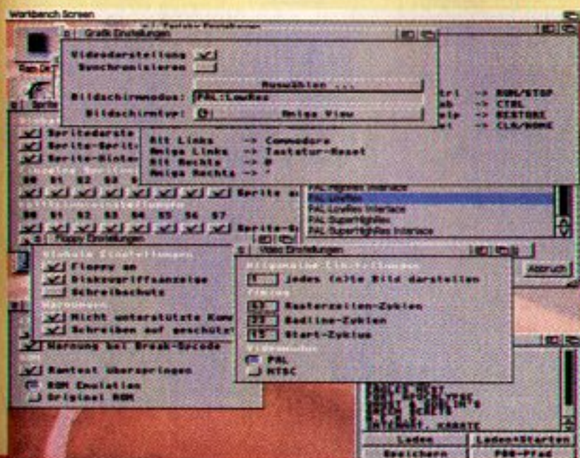
Das MagiC64-Einstellmenü
