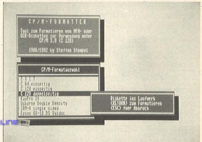
[2] Drei Modi stehen CP/M-Disketten zur Verfügung
