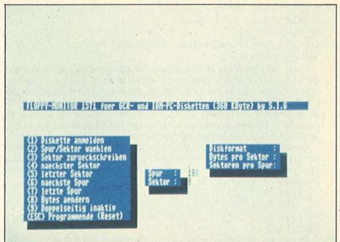
[5] Im Hauptmenü von »1571Mon« kann man zehn Funktionen aktivieren
