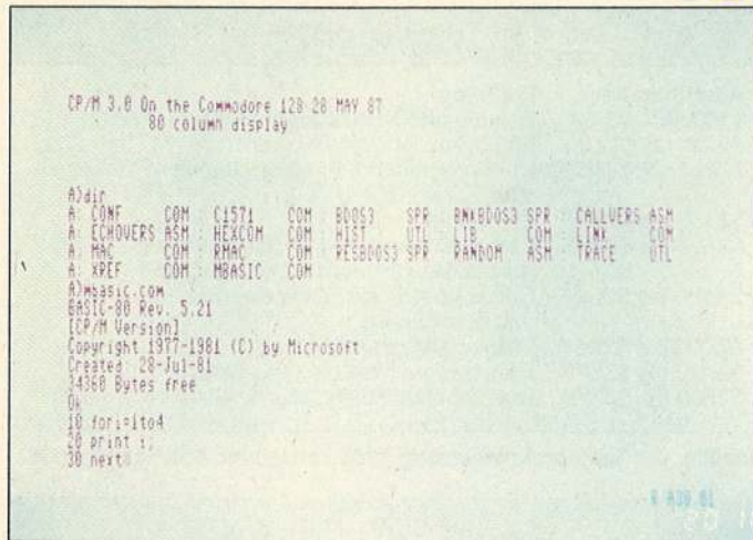
[1] Der Urvater des GWBasic der IBM-PC-kompatiblen Computer: MBasic 5.21
