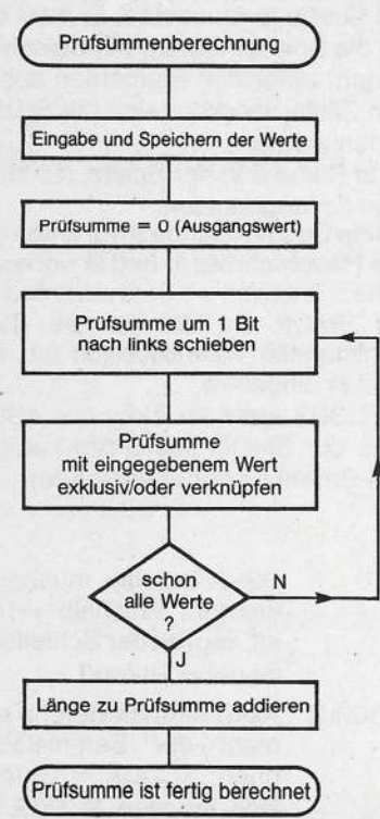
Bild 4. Das Flußdiagramm zur Prüfsummenberechnung
