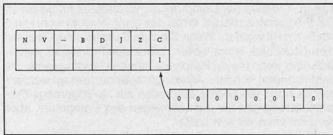
Bild 11. Das Carry-Bit als Bit 8 einer Rechenoperation
