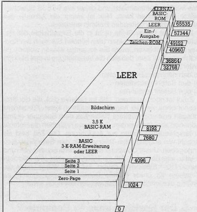
Bild 3. VC 20-Speicher (Grundversion oder mit 3-KByte-Erweiterung)
