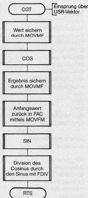
Bild 1. Flußdiagramm einer Kotangens-Funktion
