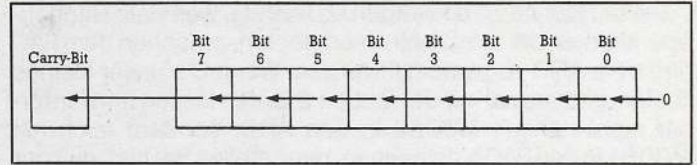
Bild 24. Wirkung des ASL-Befehls: Arithmetisches Linkschieben
