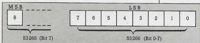
Bild 47. So sieht das 9-Bit-Register im VIC-II-Chip aus, welches die Rasterzeilen mitzählt.
