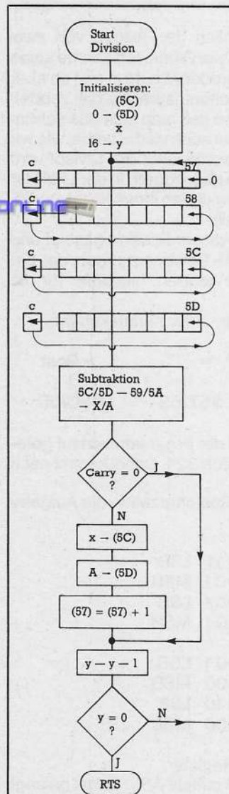
Bild 32. Flußdiagramm des Programms zur 16-Bit-Division
