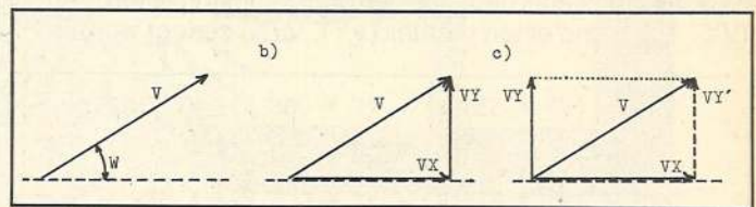
Bild 1. Vektordarstellung durch Winkel und Komponenten
