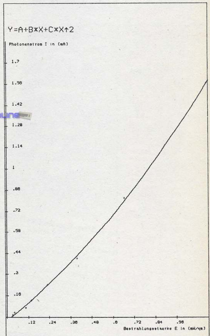
Bild 1. Die Auswertung der Meßergebnisse für die Kennlinie eines Fototransistors (mit dem Commodore-Plotter VC 1520)
