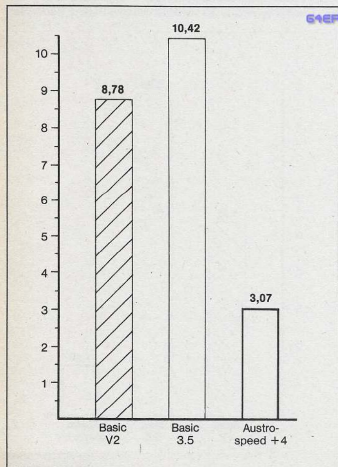
Bild 5. Das Füllen eines auf 1000 Felder dimensionierten Arrays: Immerhin dreimal schneller.
