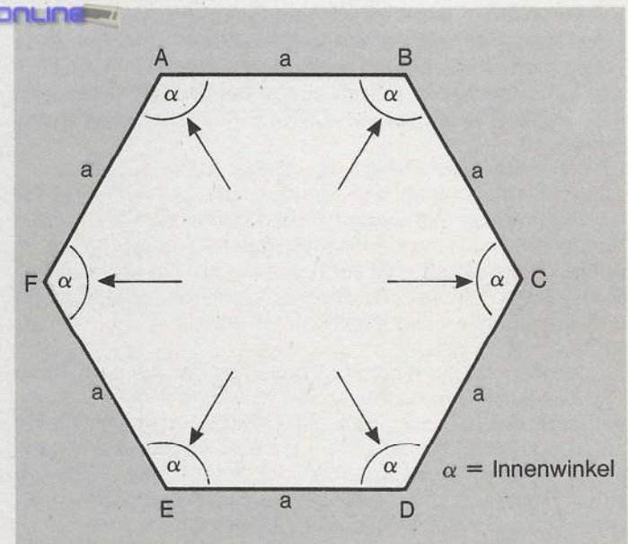
Bild 7. Regelmäßige Sechsecke weisen gleiche Innenwinkel und Kantenlängen auf
