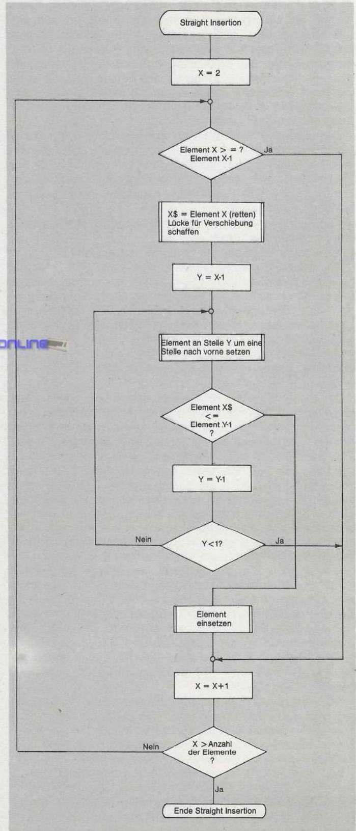
Bild 1. Das Flußdiagramm zu Straight Insertion
