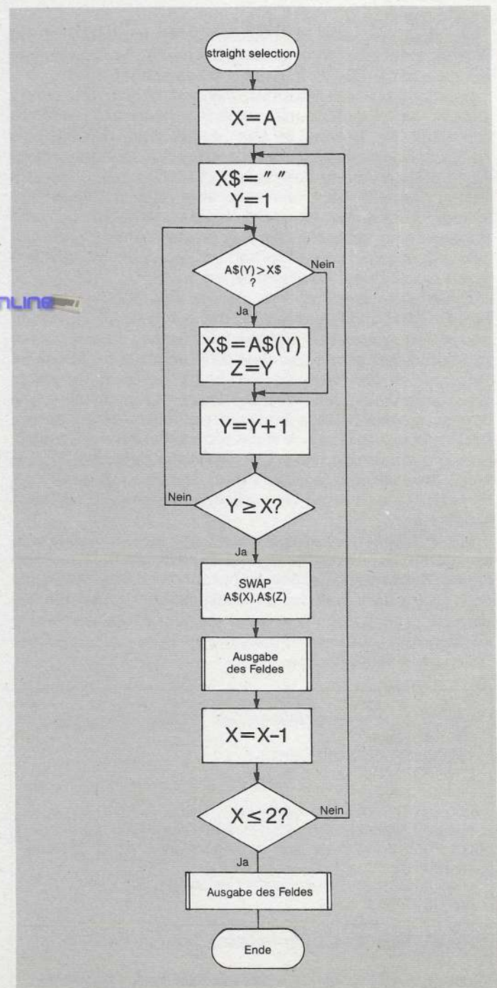
Bild 3. Straight Selection arbeitet nach dem Auswahlprinzip
