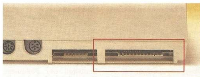
Bild 3. Der User-Port des C 64
