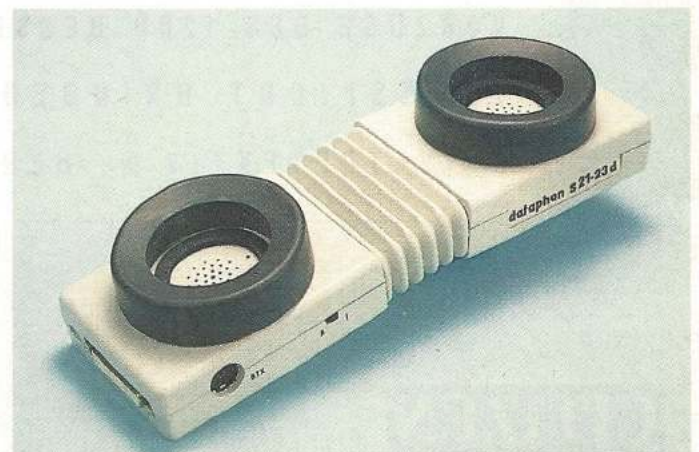
Bild 3. 1200/75-bps-Koppler mit seitlicher Anschlußbuchse für Btx-Decoder: Dataphon s21/23d (ab 350 Mark)
