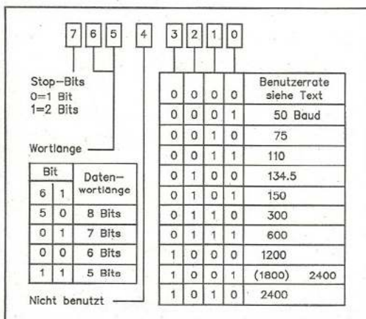
Bild 5. Die Steuerregister der RS232C
