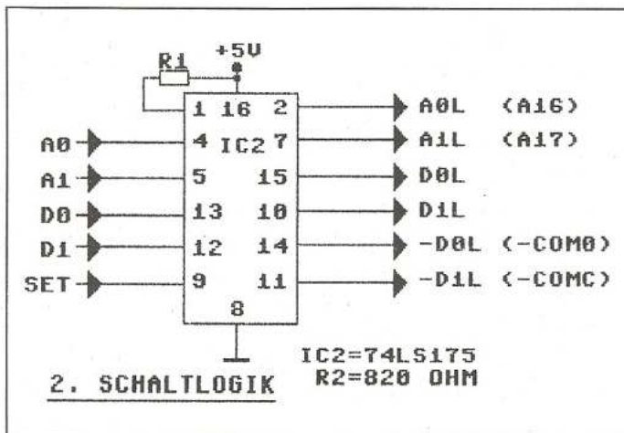
Bild 2. RAM-Schaltlogik
