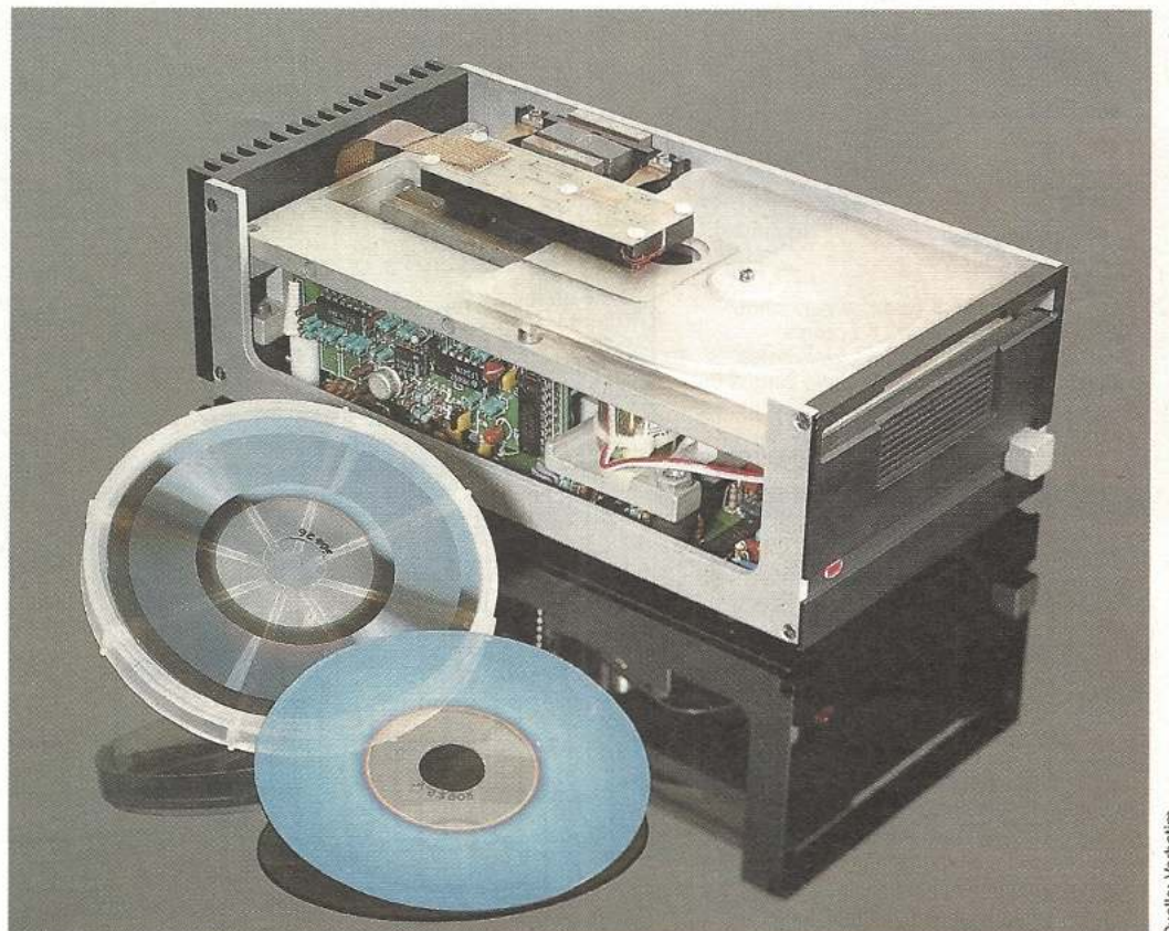
Bild 10. Ein TMO-Speicher (»Thermo Magnetic Optical«). Hierbei handelt es sich um ein System der jüngsten Generation, das vermutlich 1988 auf den Markt kommen wird. Die 3 1/2-Zoll-Platten können beliebig beschrieben werden und haben eine Speicherkapazität von 100 MByte pro Platte.
