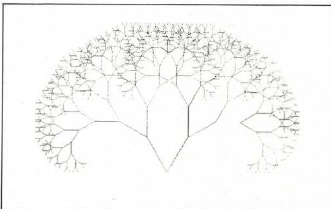
Bild 2. Ein Baum mit verändertem Winkel und Verkürzungsfaktor
