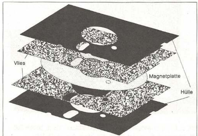
Bild 4. Schnitt durch eine handelsübliche 5¼-Zoll-Diskette
