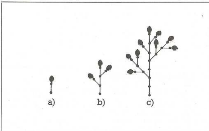
Bild 6. Die Gesetzmäßigkeit eines Baumes
