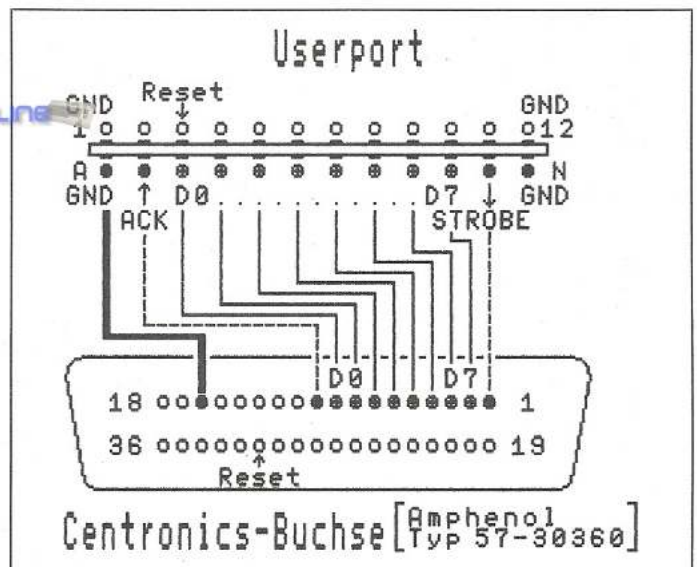
Bild 1. Verbindungskabel User-Port/Centronics-Schnittstelle
