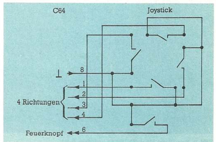
Bild 1. Nach diesem Schema werden die Joystickports abgefragt
