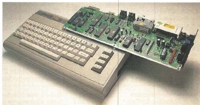
Bild 1. Der neue C 64 und dessen überarbeitete »Innereien«
