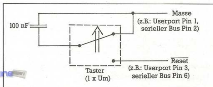
Bild 1. So schließen Sie den »Spezial-Reset-Taster« an
