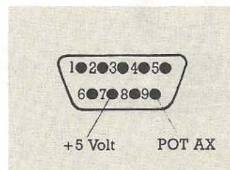
Bild 4. Anschlußbelegung des Control-Ports 1
