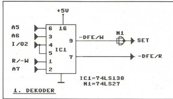
Bild 5. RAM-Decodierung
