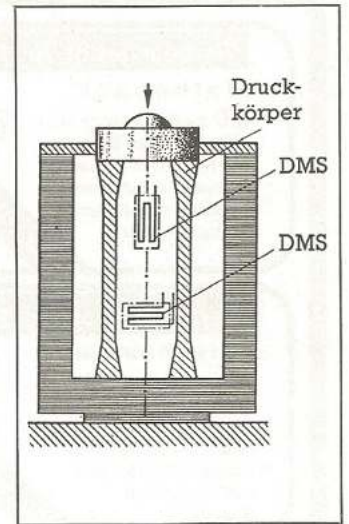
Bild 4. Eine Verwendung von Dehnungsmeßstreifen (DMS)
