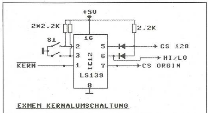
Bild 11. Betriebssystem Umschaltlogik
