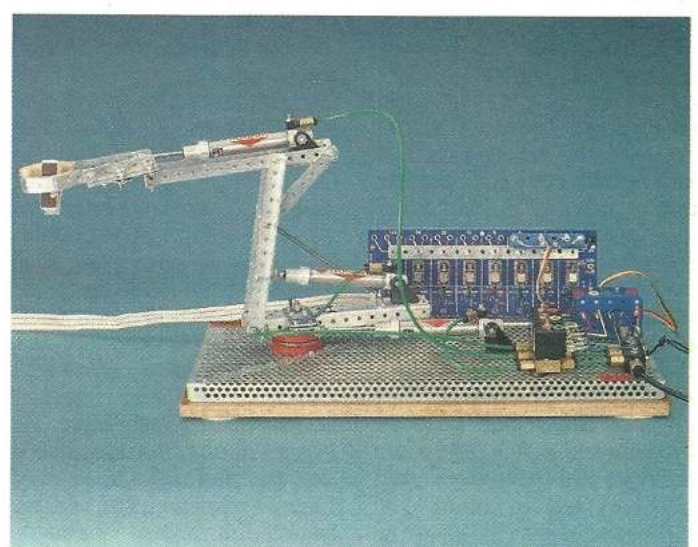
Bild 3(+3a). Beim »Robby I« werden industriemäßige Pneumatikzylinder verwendet. Der Roboter kann auch über auswechselbare Nockenwalzen gesteuert werden (oben).
