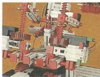
Bild 6(+6a). Beim »Trainingsroboter« sind Spindeltrieb und Gabellichtschranken deutlich zu erkennen (unten)
