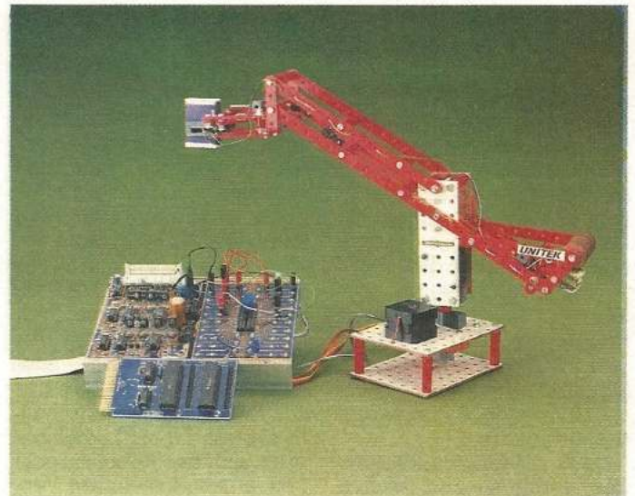
Bild 5(+5a). Der »Unitek-Roboter« kann sich mit seinen Schrittmotoren erstaunlich schnell bewegen. Im Test ist es der einzige C 64-Roboter mit einer Fühleinrichtung im Greifer (unten).
