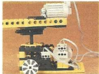
Bild 4(+4a). Bei dem »Lego-Roboter« kontrolliert der C 64 die Drehbewegung über einen Optosensor und eine Zählscheibe (unten abgenommen und umgedreht).
