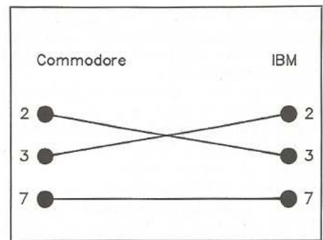
Bild 6. So müssen die Kabel verdrahtet sein, wenn Sie den C 64 an einen IBM-PC anschließen
