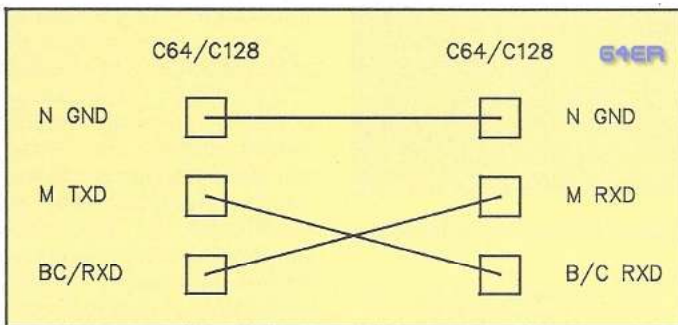
Bild 1. Verbindung von C 64 — C 64 über Nullmodem
