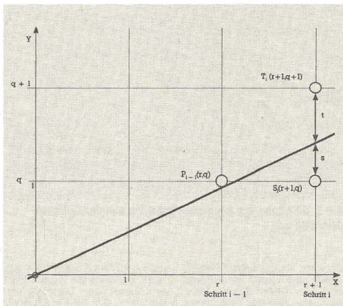
Bild 2. Der Besenham-Linialalgorithmus basiert auf der Ermittlung der Abstände s und t von der Ideallinie
