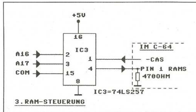
Bild 7. RAM-Steuerung
