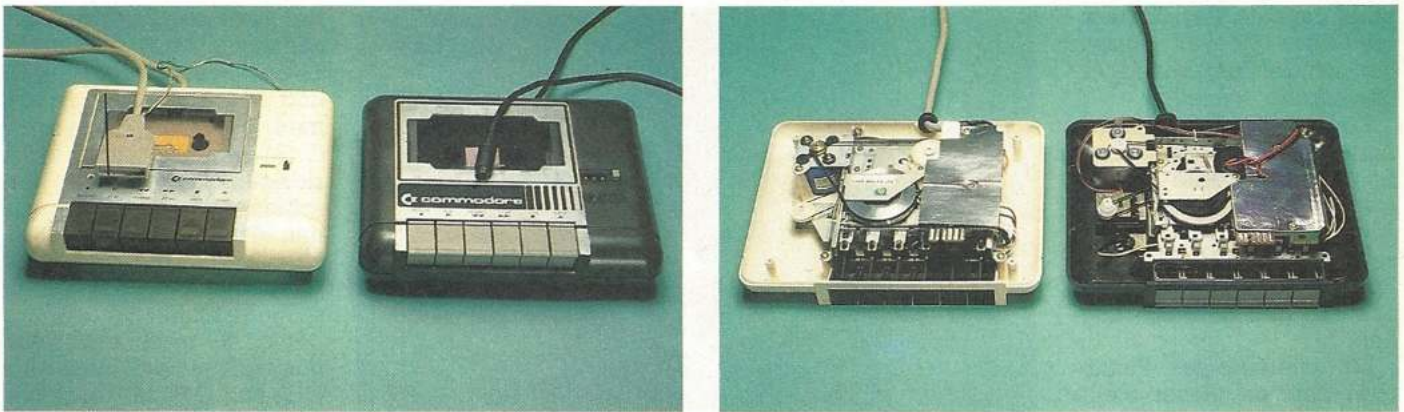
Bild 3.1 und 3.2. Die beiden Datasetten von Commodore sind bis auf die Stecker und unwesentliche Details absolut identisch. Die Laufwerksmechanik ist von einem jeweils anderen Hersteller und wurde geringfügig modifiziert.
