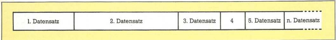
Bild 1. Der Aufbau einer sequentiellen Datei. Die Datensätze können unterschiedlich lang sein und hängen direkt hintereinander.
