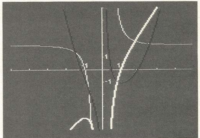
Bild 3a. Das komplette Ergebnis einer Kurvendiskussion nach dem DISCUSS-Befehl (Grafik).
