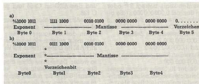
Bild 3. a) 1985,125 im FLPT- und b) im MFLPT-Format
