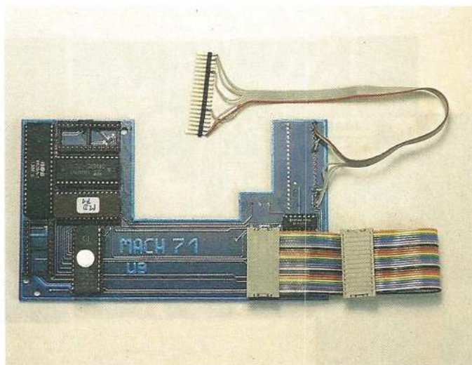
Bild 2. Der Floppy-Speeder für die 1571
