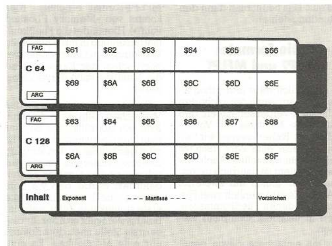
Bild 4. Orte und Aufbau der beiden Fließkomma-Akkumulatoren im C 64 und im C 128
