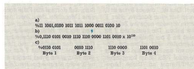
Bild 5. a) errechneter Nachkommaanteil b) Normalisieren c) GRDFAK im MFLPT-Format
