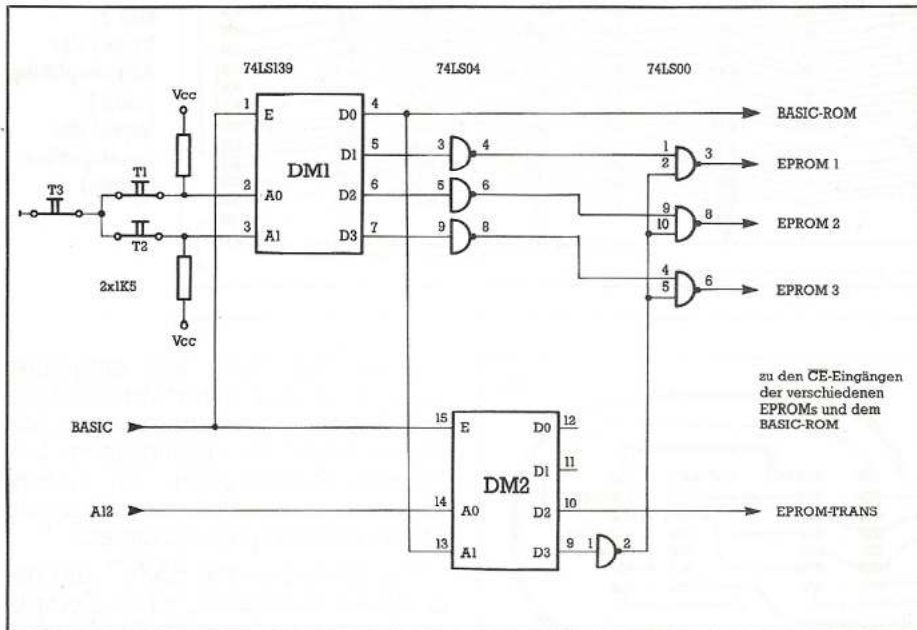
Bild 2. Zusatzschaltung zur Steuerung der verschiedenen EPROMs und dem Basic-ROM
