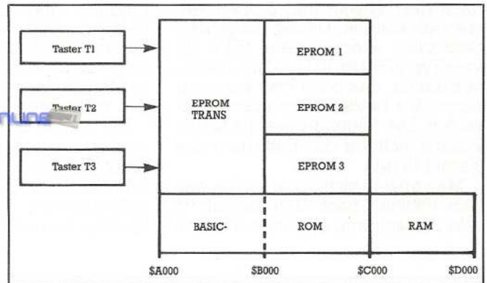
Bild 1. Speicherorganisation mit Zusatzschaltung
