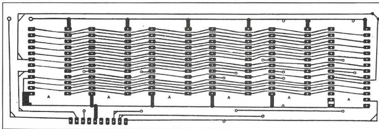
Bild 3. Layout der Adapterplatine (oben); Layout der Zusatzplatine (unten)
