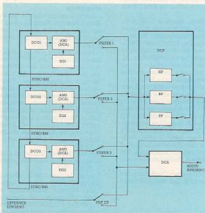
Bild 1. Blockschema des SID
