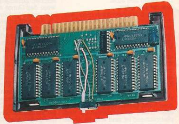
Bild 2. 16-KByte-Erweiterung mit eingebautem Umschalter, geöffnet.
