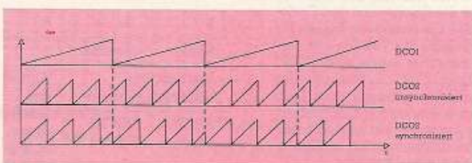
Bild 2. Die Synchronisation
